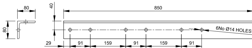
TPL-B-1 - EA 80x80x8 Scale 1:10
